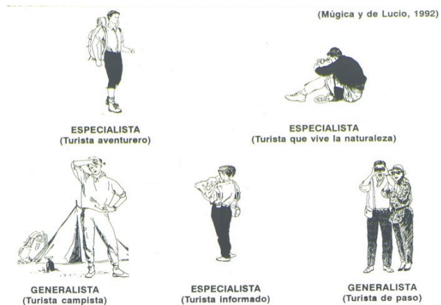
Figura 4. Perfiles de visitantes de parques nacionales en España a principios de los años noventa.
