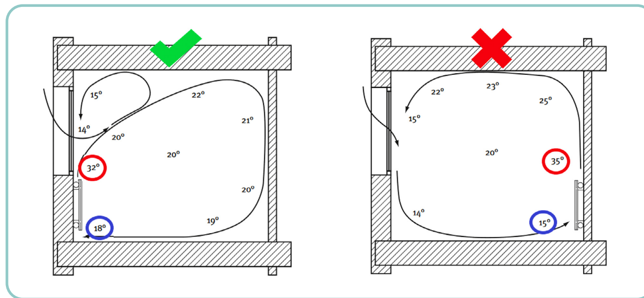
Distribución de la temperatura en función de la colocación del radiador. A la izquierda se pueden ver las ventajas de colocarlo bajo la ventana.
